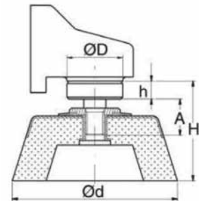
S) Schleiftopf
