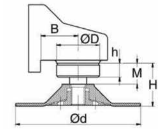
F) Schleifteller
